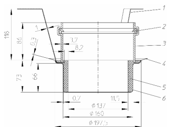
Рис. 6. Противопожарная муфта HL870 для кровельной воронки HL62.1Н/1.
