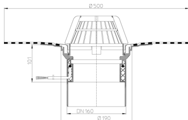
Рис. 3. Кровельная воронка с электрообогревом для внутреннего водостока HL62.1H/2.
