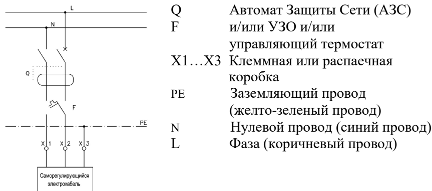
Рис. 5. Схема подключения электрообогрева кровельной воронки HL62.1Н к электрической сети.
