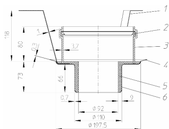
Рис. 5. Противопожарная муфта HL850 для кровельной воронки HL62.1Н/7.
