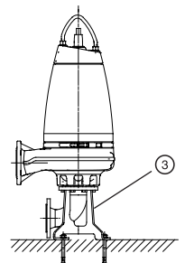
Вертикальная сухая установка
