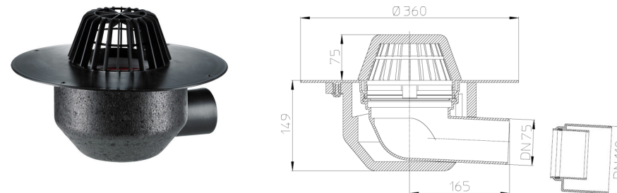
Рис. 1. Кровельная воронка HL64F.
