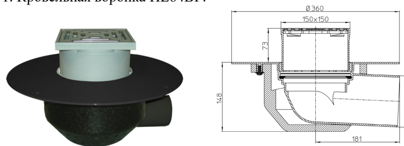
Рис. 1. Кровельная воронка HL64BF.
