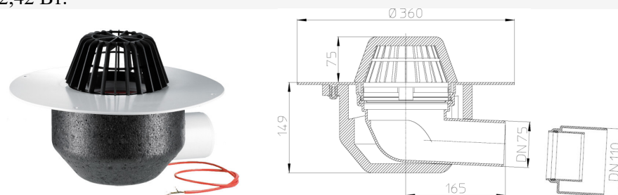
Рис. 1. Кровельная воронка HL64.1P.
