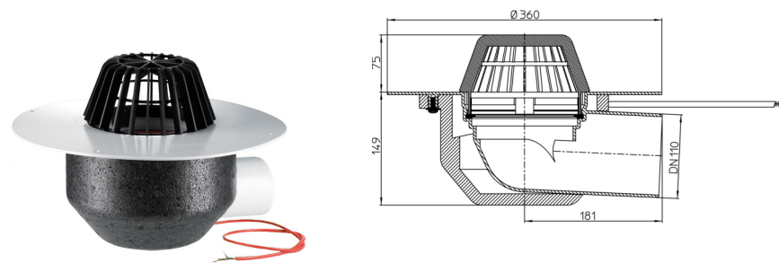
Рис. 2. Кровельная воронка HL64.1P/1.
