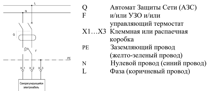
Рис. 2. Схема подключения комплекта электрообогрева HL155 к электрической сети.
