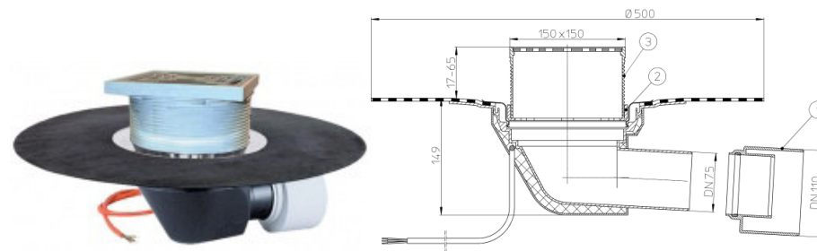
Рис. 1. Кровельная воронка с электрообогревом HL64.1BH
