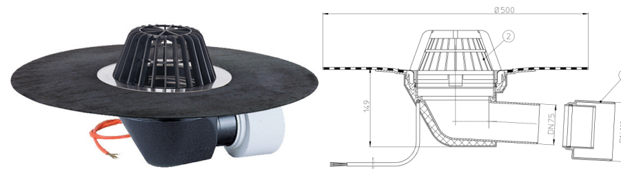
Рис. 1. Кровельная воронка с электрообогревом HL64.1H
