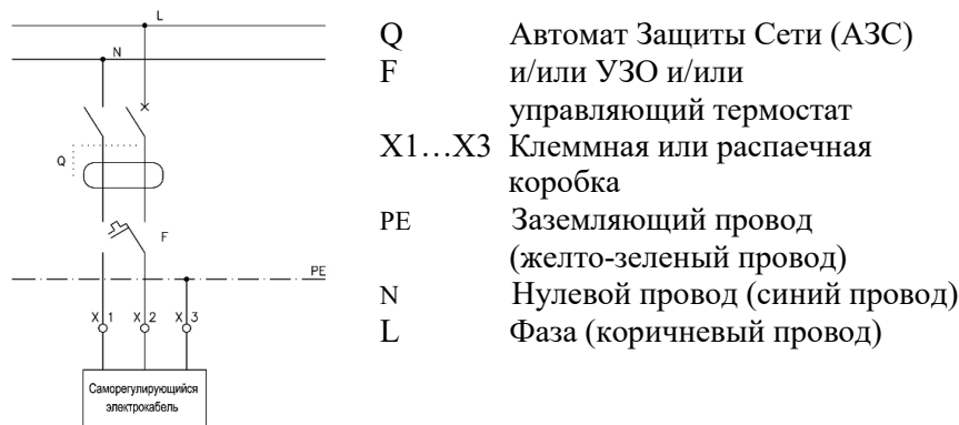
Рис. 2. Схема подключения электрообогрева кровельной воронки HL64.1H к электрической сети.
