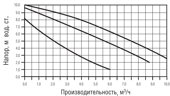
Диаграммы характеристик насоса WCP 25-100G, WCP 32-100G
