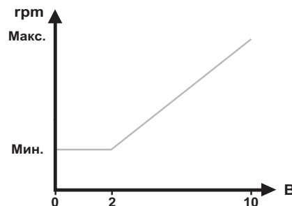
Рис. 61 Зависимость скорости насоса от установленного значения сигнала 0–10 В
