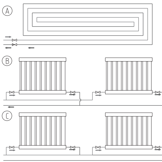
Рис. 41 Настройка режима работы
