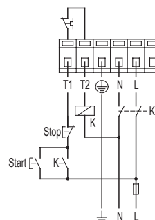
Рис. 19 Однофазный
