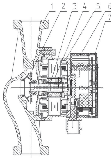
Рис. 31 Насос MASTER S
