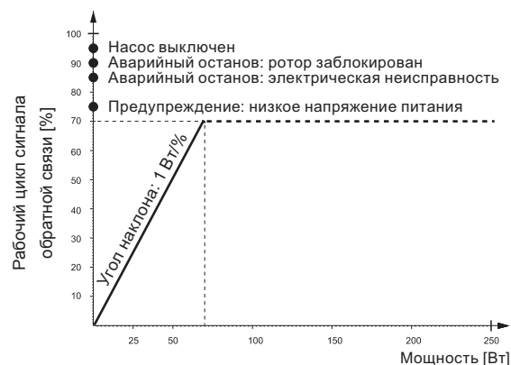
Рис. 30 Профиль ШИМ-сигнала обратной связи
