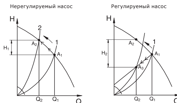
Рис. 28 Изменение положения рабочей точки регулируемого и нерегулируемого насоса
