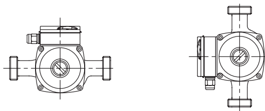
Рис. 8 Возможная ориентация вала
