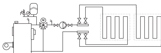
Рис. 6 Система «тёплых полов»
