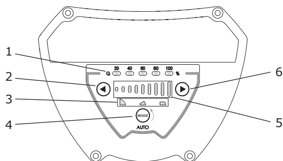
Рис. 45 Элементы панели управления
