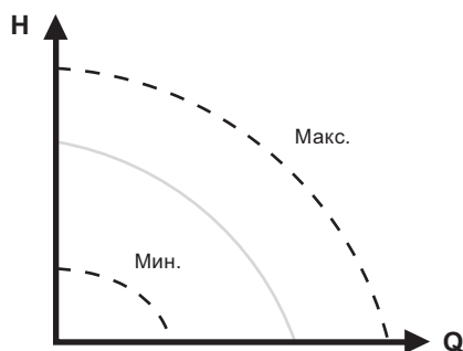
Рис. 55 Максимальная и минимальная характеристики
