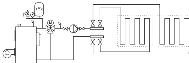
Рис. 27 Система «тёплых полов»
