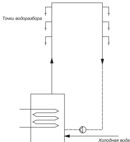
Рис. 12 Одноконтурная схема контура рециркуляции горячей воды
