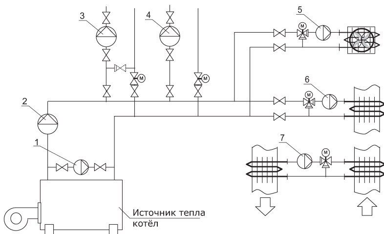
Рис. 35 Схема системы отопления
