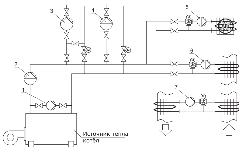
Рис. 15 Схема системы отопления и теплоснабжения
