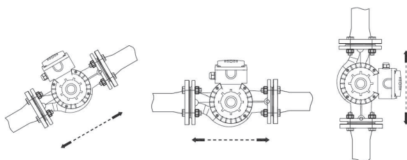
Рис. 63 Варианты монтажа
