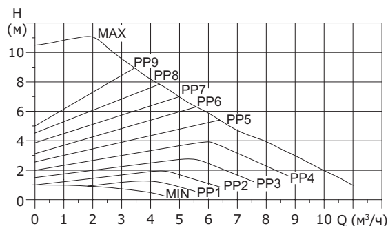
Рис. 42 Кривые режима управления пропорционального изменения давления
