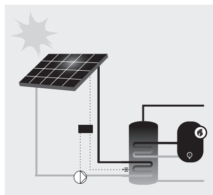
Рис. 54 Функциональная схема системы отопления на основе использования энергии солнца
