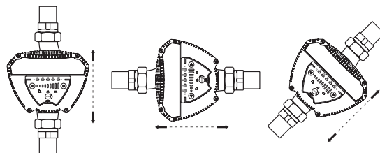
Рис. 37 Допустимое расположение вала насоса
