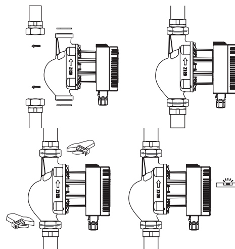
Рис. 39 Монтаж насоса
