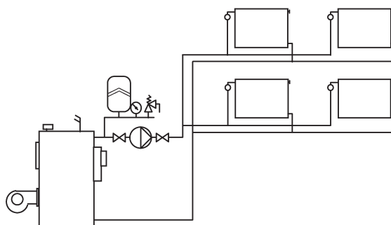
Рис. 26 Двухтрубная система отопления
