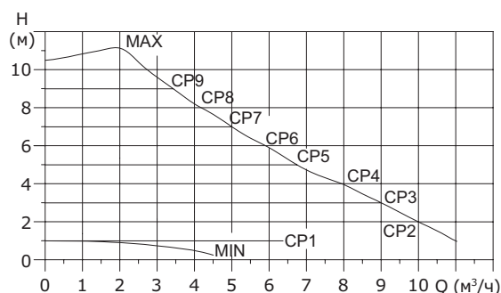
Рис. 43 Кривые режима управления с постоянным значением давления.
