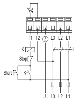
Рис. 20 Трехфазный без нейтрального провода
