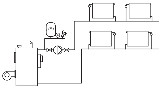
Рис. 25 Однотрубная система отопления
