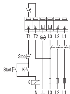
Рис. 21 Трехфазный с нейтральным проводом
