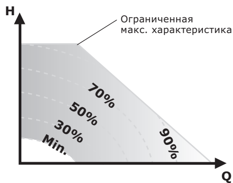
Рис. 60 Ограничения по мощности и давлению, влияющие на максимальную характеристику
