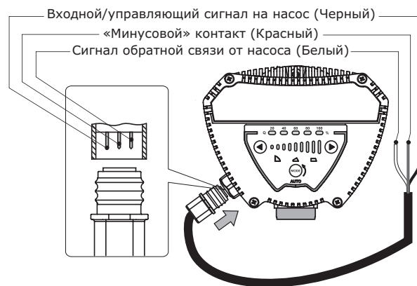
Рис. 46 Схема подключения ШИМ-сигнала
