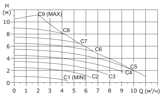
Рис. 44 Кривые режима управления при фиксированной частоте вращения
