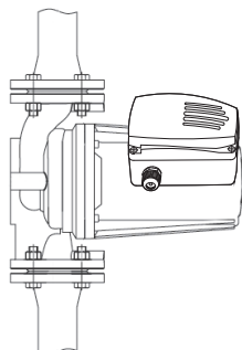
Рис. 17 Положение вала электродвигателя
