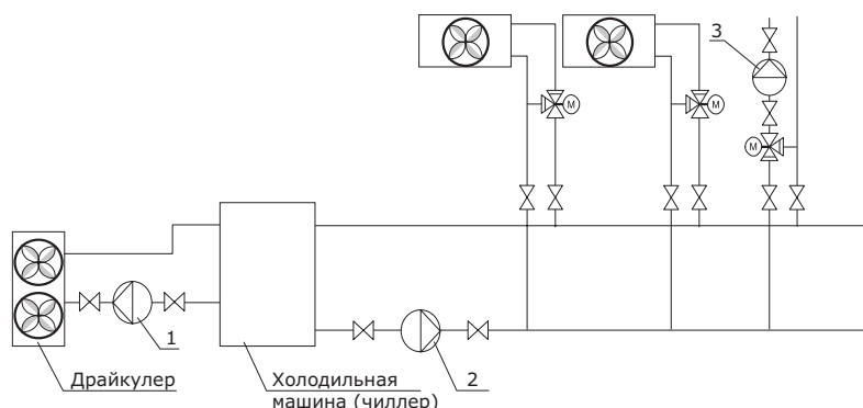
Рис. 16 Схема системы охлаждения и кондиционирования воздуха
