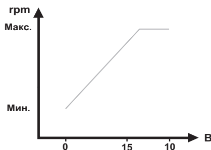
Рис. 62 Зависимость скорости насоса от установленного значения сигнала 4–20 мА
