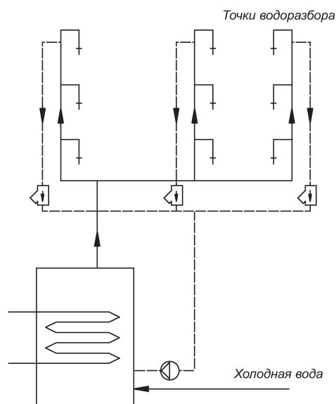
Рис. 13 Многоконтурная схема рециркуляции горячей воды
