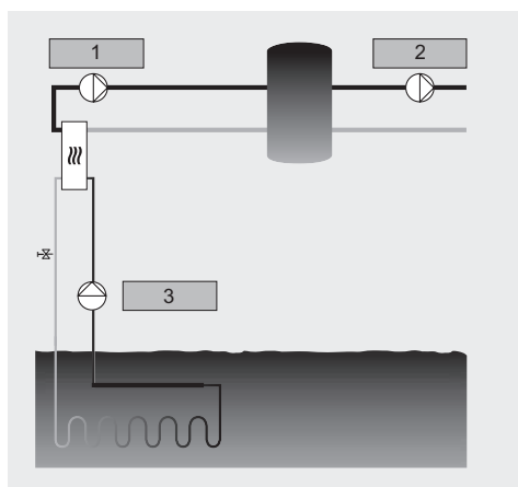
Рис. 53 Функциональная схема системы отопления на основе использования теплоты грунта
