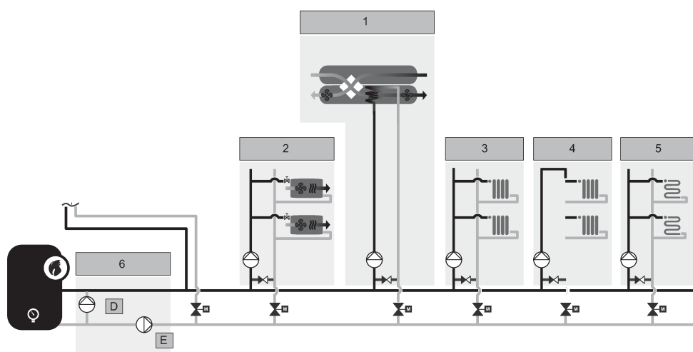
Рис. 51 Функциональная схема системы отопления в коммерческом здании
