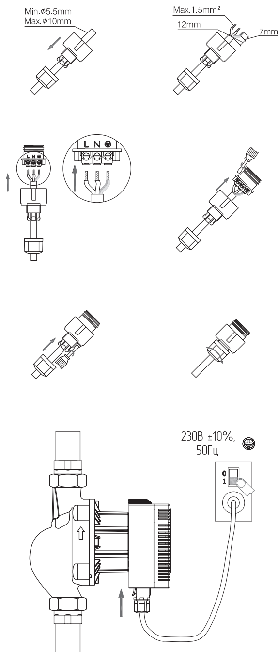
Рис. 40 Электроподключение насоса
