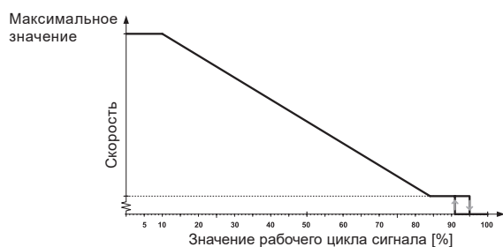
Рис. 29 Профиль управляющего ШИМ-сигнала
