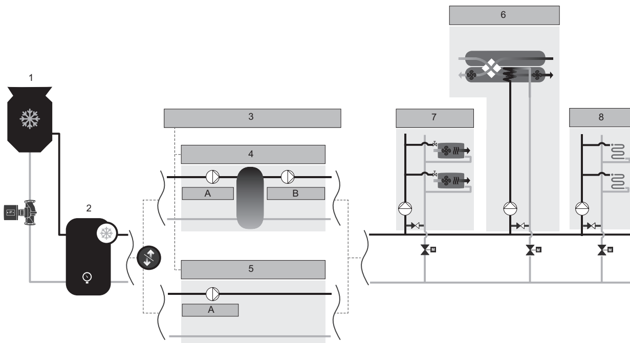
Рис. 52 Функциональная схема системы охлаждения в коммерческом здании
