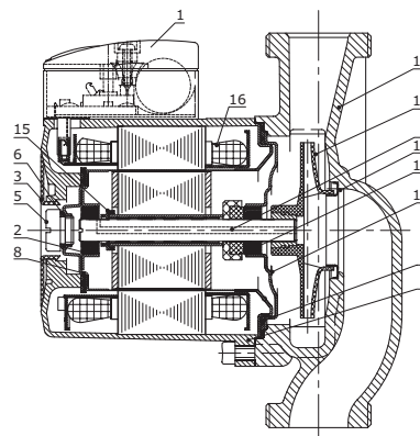
Рис. 7 Трехскоростной насос BASIC S
