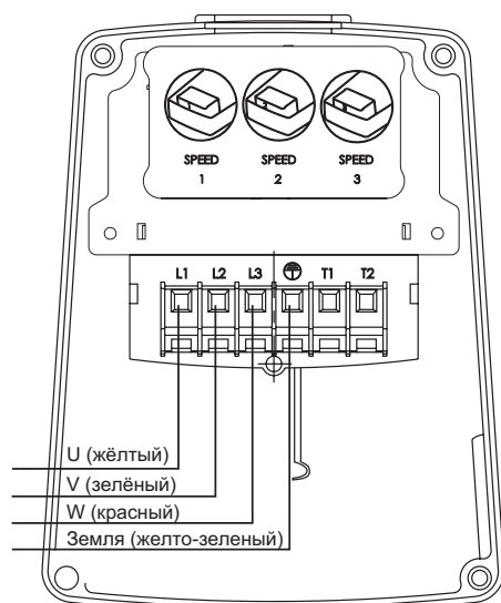
Рис. 22 Модуль переключения частоты вращения
