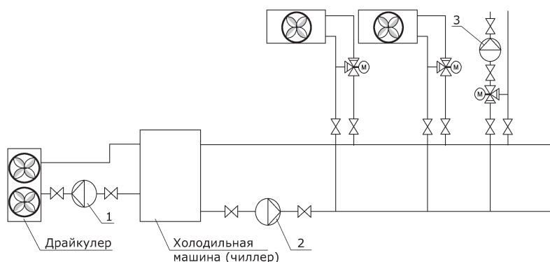
Рис. 36 Схема системы кондиционирования воздуха
