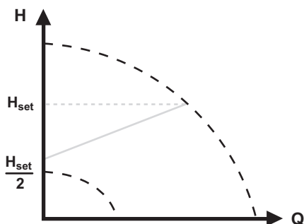
Рис. 56 Регулирование по пропорциональному давлению
