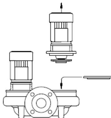
Fig. 4 De blindflens bevestigen
