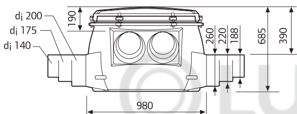
Теплоизолированный колодец 1000
