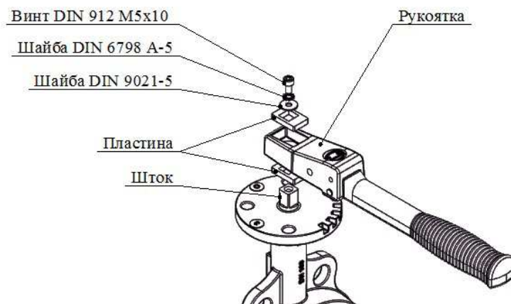
Рисунок 1 – Установка рукоятки
