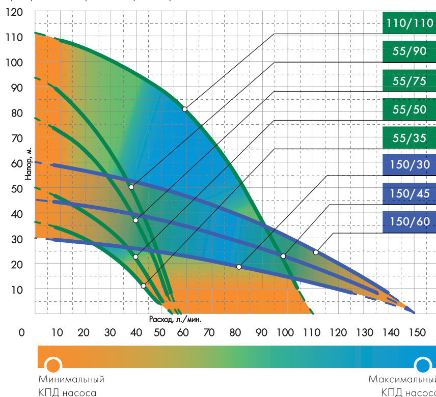
График напорных характеристик*:
