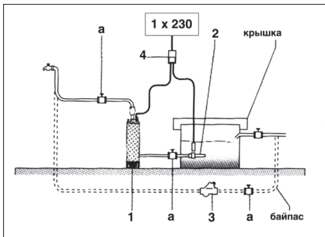
Рис. 2 1 – насос 2 – приемный клапан 3 – обратный клапан 4 – реле давления a – шаровый кран
