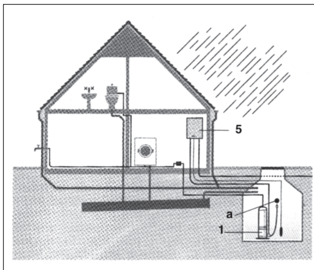
Рис. 1 1 – насос 5 – модуль управления Presscontrol PC15 a – шланг с поплавком
