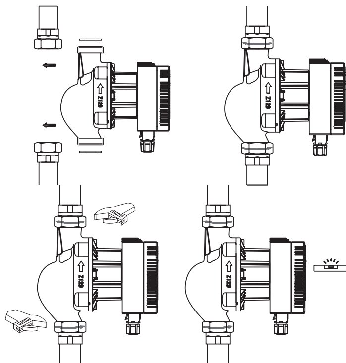
Рис. 3 Монтаж насоса
