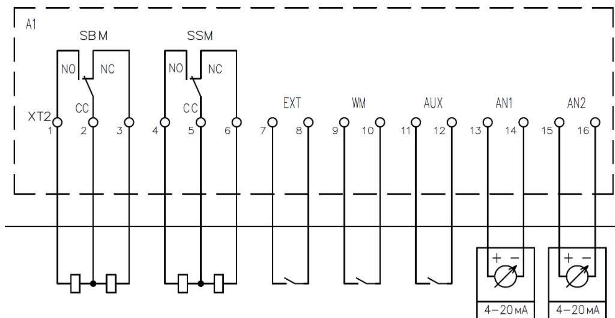
Рис. 3 Подсоединения сетевых контактов и клеммных колодок
