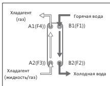
Рисунок(1) Испаритель
