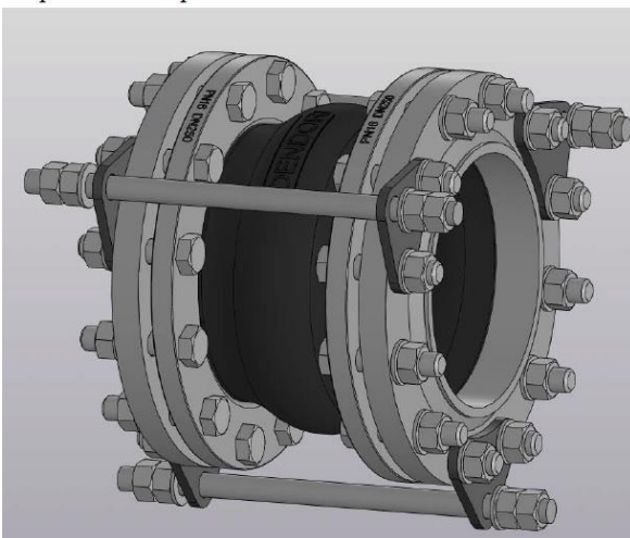
Ограничитель растяжения
