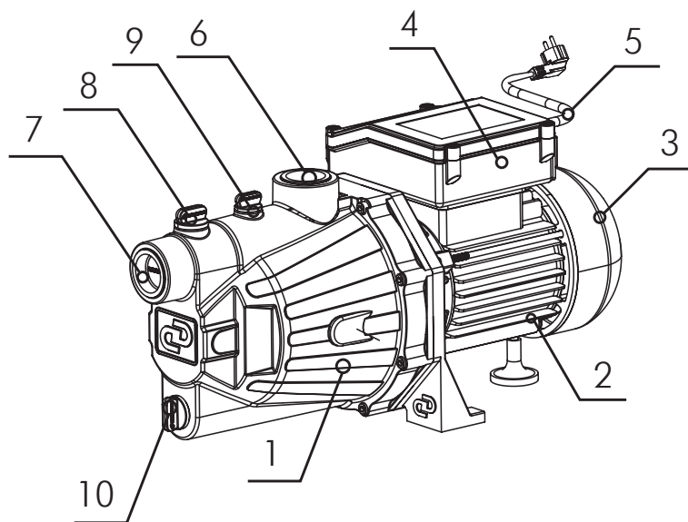
Рисунок 2 Общий вид поверхностного насоса «ДЖАМБО» (П, Ч)
