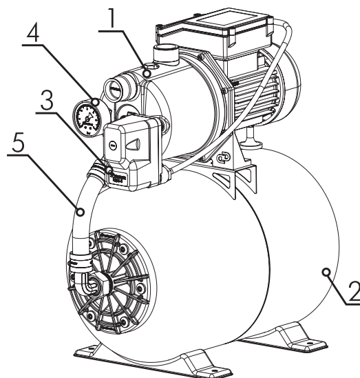
Рисунок 5 Общий вид насоса-автомата «ДЖАМБО» (Н)
