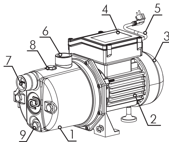
Рисунок 3 Общий вид поверхностного насоса «ДЖАМБО» (Н)
