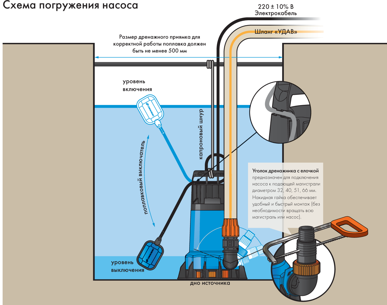
Рисунок 4 (на примере изображен насос «ДРЕНАЖНИК» 350/17).
