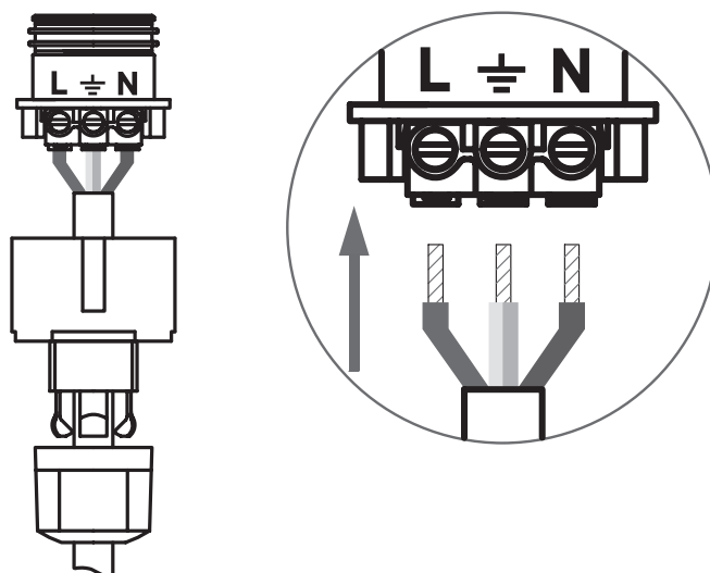
Рис. 8 Схема подключения насоса
