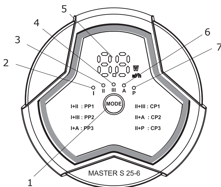
Рис. 12 Панель управления
