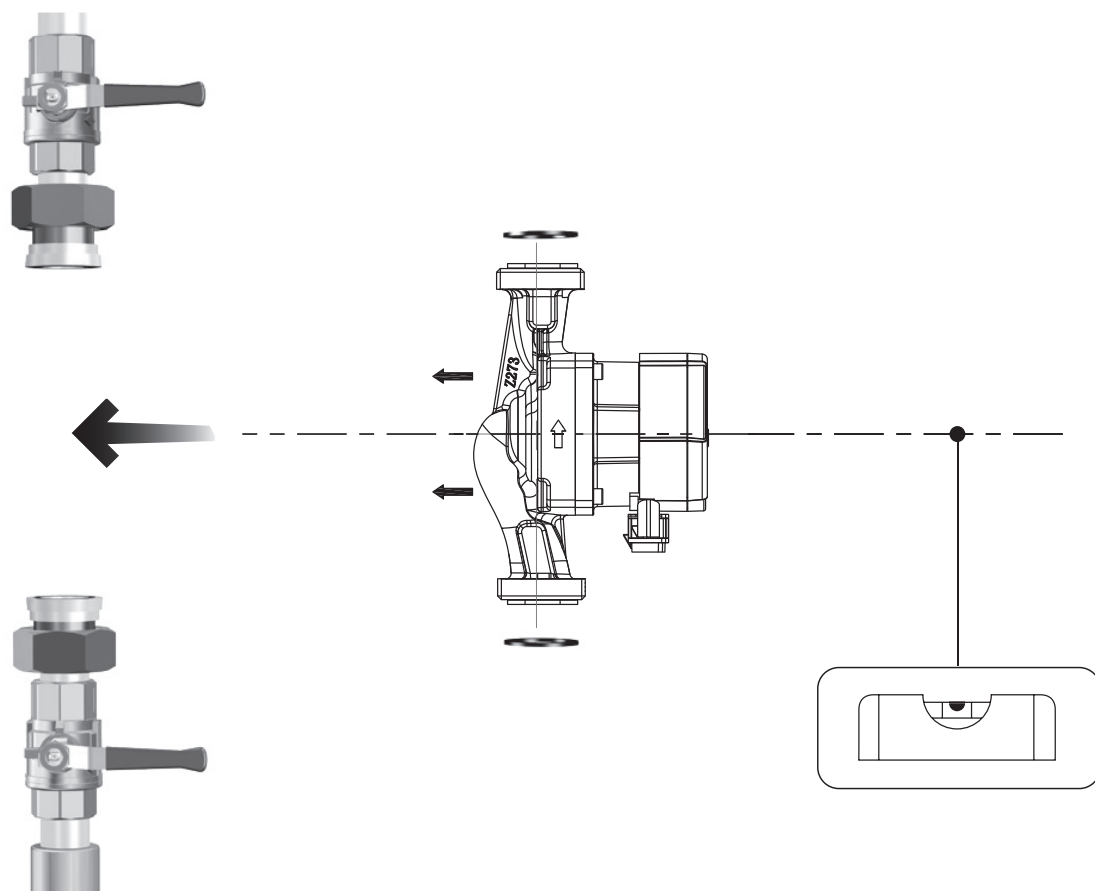
Рис. 3 Монтаж насоса
