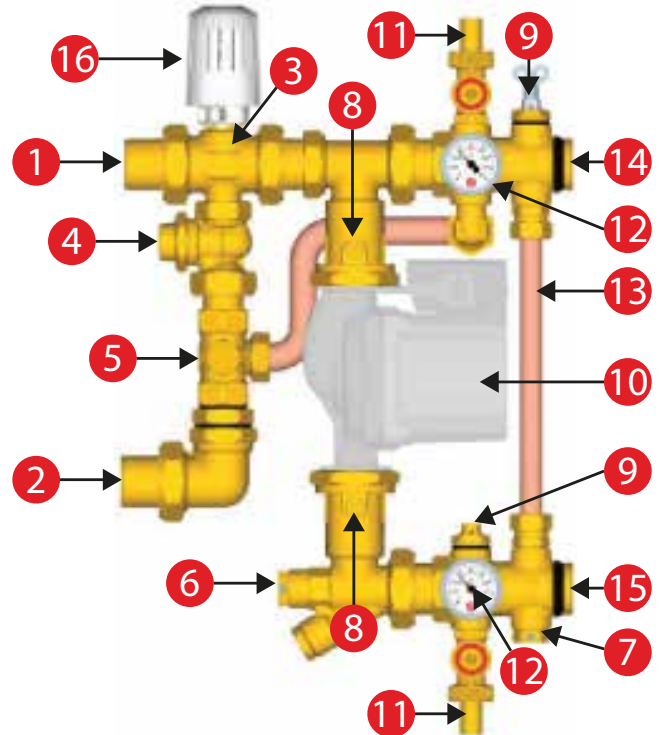
Составные элементы узла R557RY043
