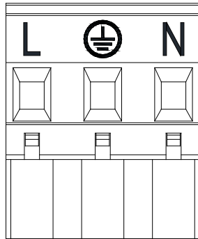
Abbildung 6: Abnehmbares Klemmenbrett der Versorgung
