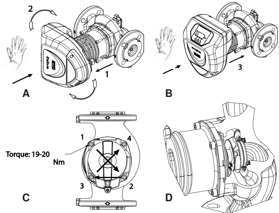
Fig 2: Monteringsanvisningar för motorhuvud
