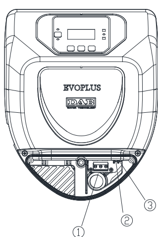
Сх. 4: Электрические соединения (вид спереди)
