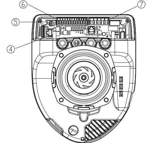
Resim 5: Elektrik bağlantıları (arka)
