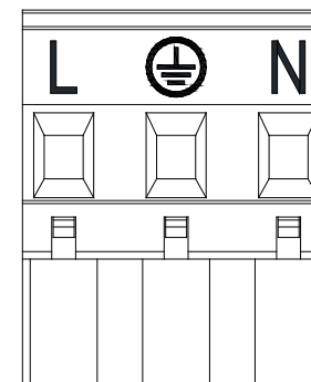
6. ábra: kivehető sorkapocs tábla a tápfeszültséghez
