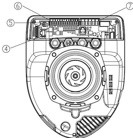
Сх. 5: Электрические соединения (вид сзади)
