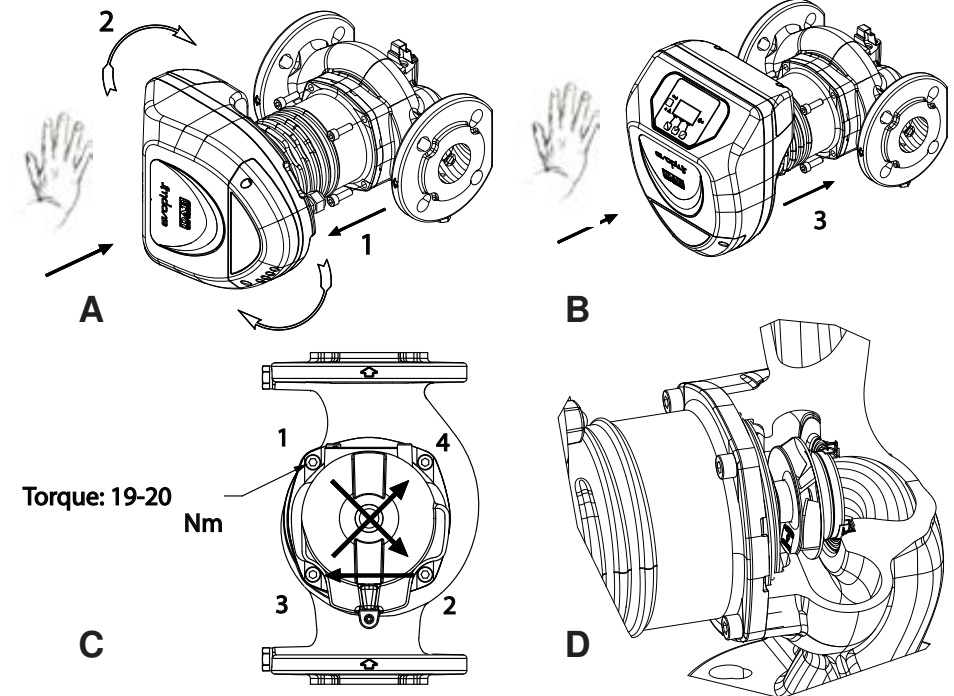
Afbeelding 2: Montage-instructies motorblokken
