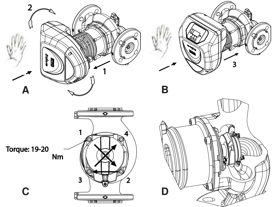
Resim 2: Motor kafaları montaj talimatları
