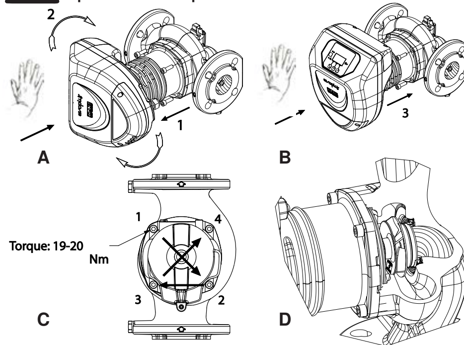
Figure 2: Instrucțiuni de montare capete motor
