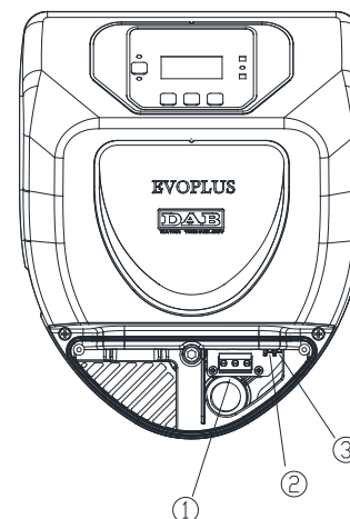
Abbildung 4: Elektroanschlüsse (Frontseite)
