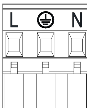
Схема 6: Изводи терминал захранване
