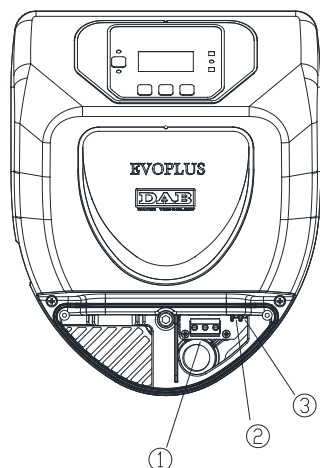
Rys. 4: Podłączenia elektryczne (przód)
