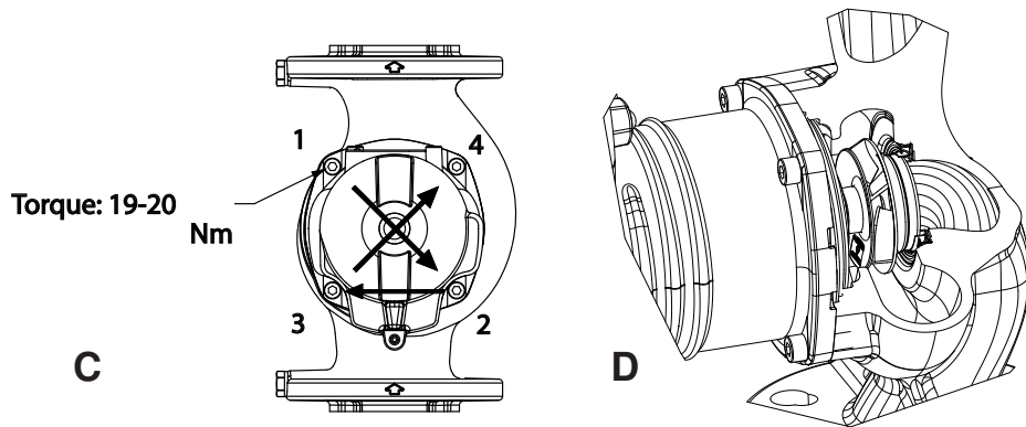
2. sz. ábra: Motortestek szerelési utasítása
