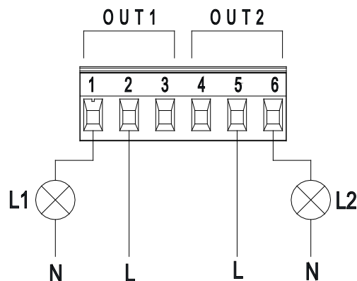
Kuv. 9: 6-napainen ulosvedettävä riviliitin: esimerkki lähtöjen kytkennästä
