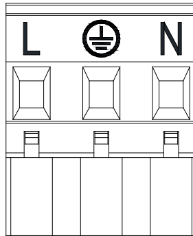
Figura 6: Morsettiera estraibile di alimentazione
