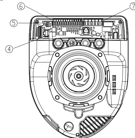
Kuv. 5: Sähköliitännät (taka)
