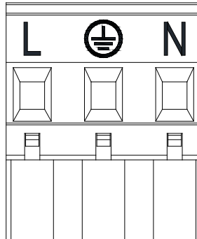
Obr. 6: Vyjímatelná svorkovnice napájení
