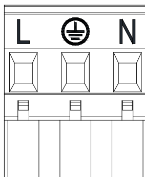
Slika 6: Snemljiva priključna sponka za priključitev napajanja
