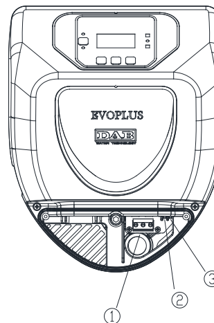
Kuv. 4: Sähköliitännät (etu)
