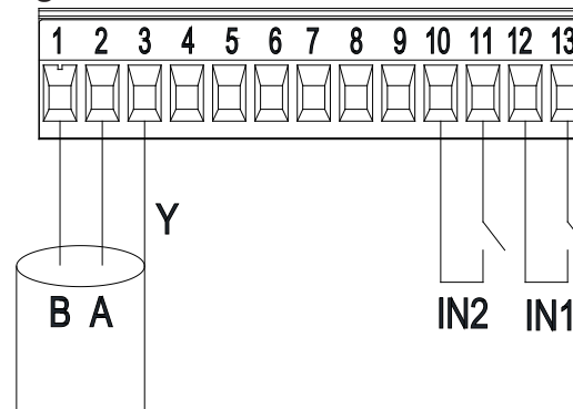
Figura 7: Barra de terminais extraível 13 pólos entradas digitais e MODBUS
