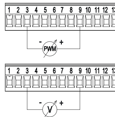
Сх. 8: Съёмная клеммная колодка 13 полюсов: входы 0-10 В и ШИМ
