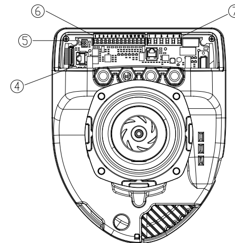
Fig. 5: Elanslutning (baksida)
