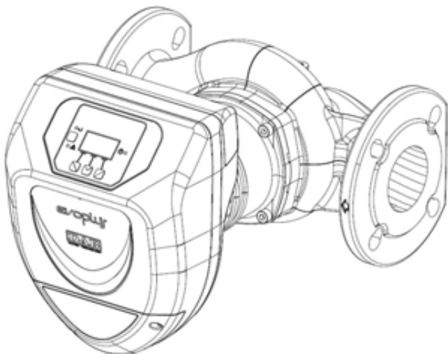
Fig. 3: Installation på horisontella ledningar
