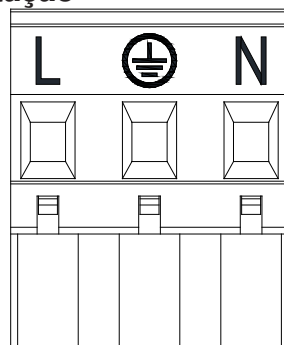
Figura 6: Barra de terminais extraível de alimentação
