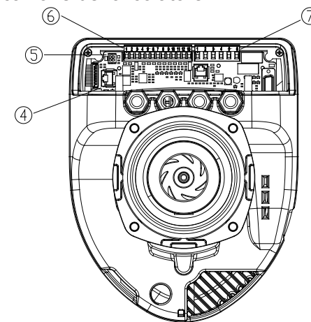
Figura 5: Connessioni elettriche (retro)
