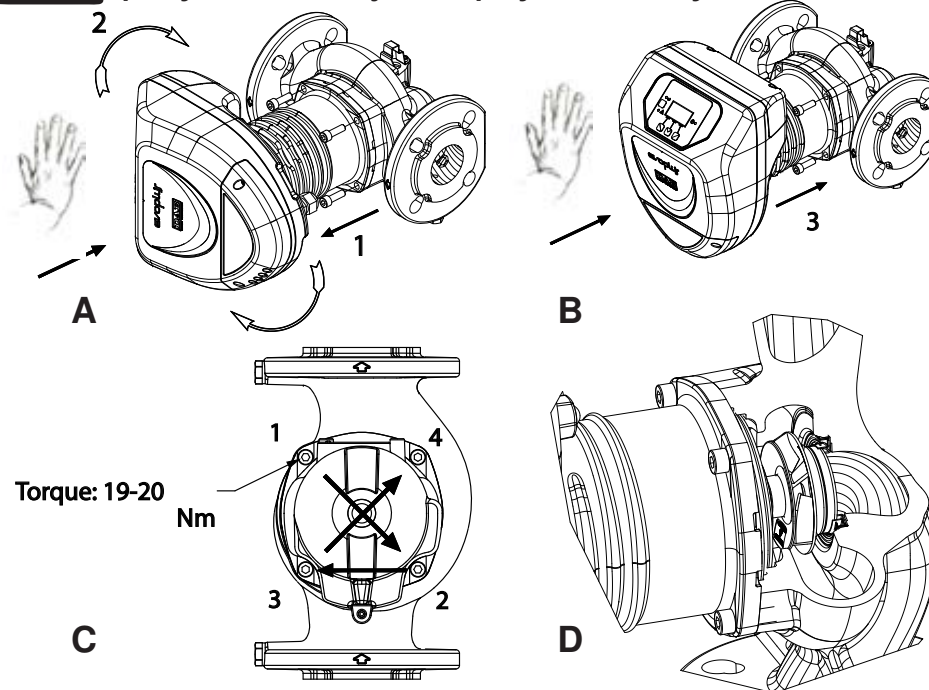
Rys. 2: Instrukcja montażu głowic silnika
