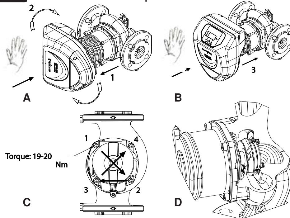
Figura 2: Instrucciones de montaje cabezales del motor
