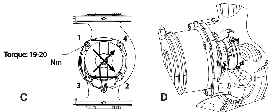
Εικόνα 2: Οδηγίες για την συναρμολόγηση των κεφαλών του κινητήρα
