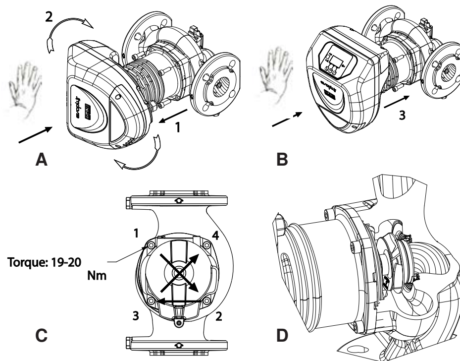
Attēls 2: Dzinēja galviņu montāžas instrukcijas
