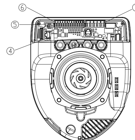
Схема 5: Електрически връзки (изглед отзад)
