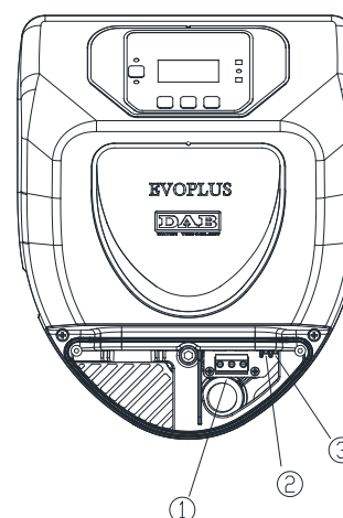
Схема 4: Електрически връзки (изглед отпред)
