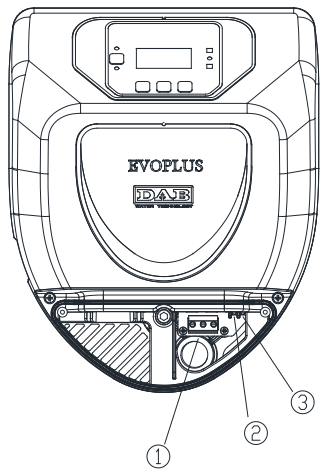
Afbeelding 4: Elektrische aansluitingen (voorzijde)
