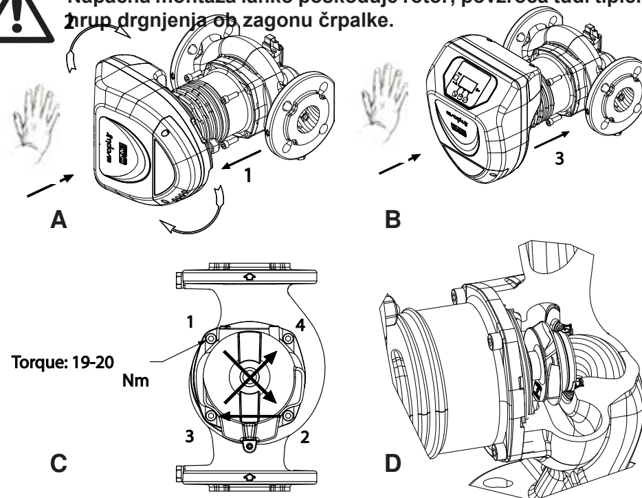
Slika 2: Navodilo za montažo glave motorja
