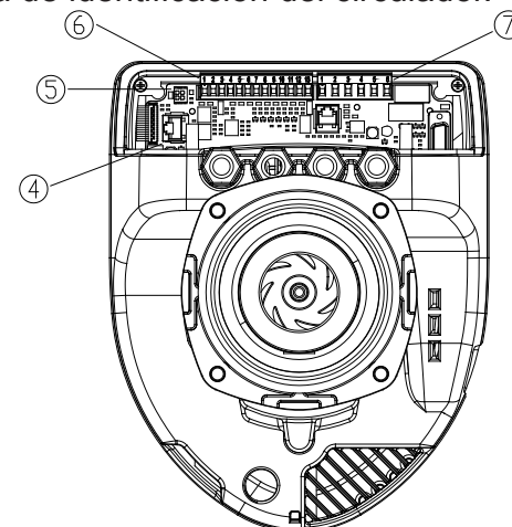
Figura 5: Conexiones eléctricas (parte posterior)
