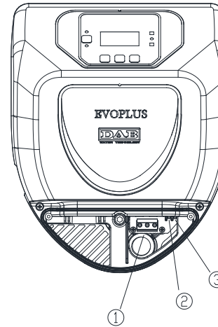
Resim 4: Elektrik bağlantıları (ön)
