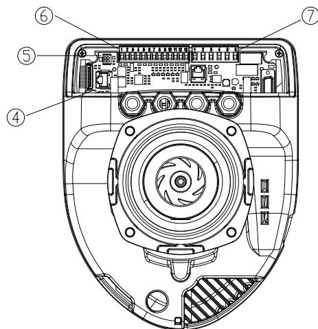
Rys. 5: Podłączenia elektryczne (tył)
