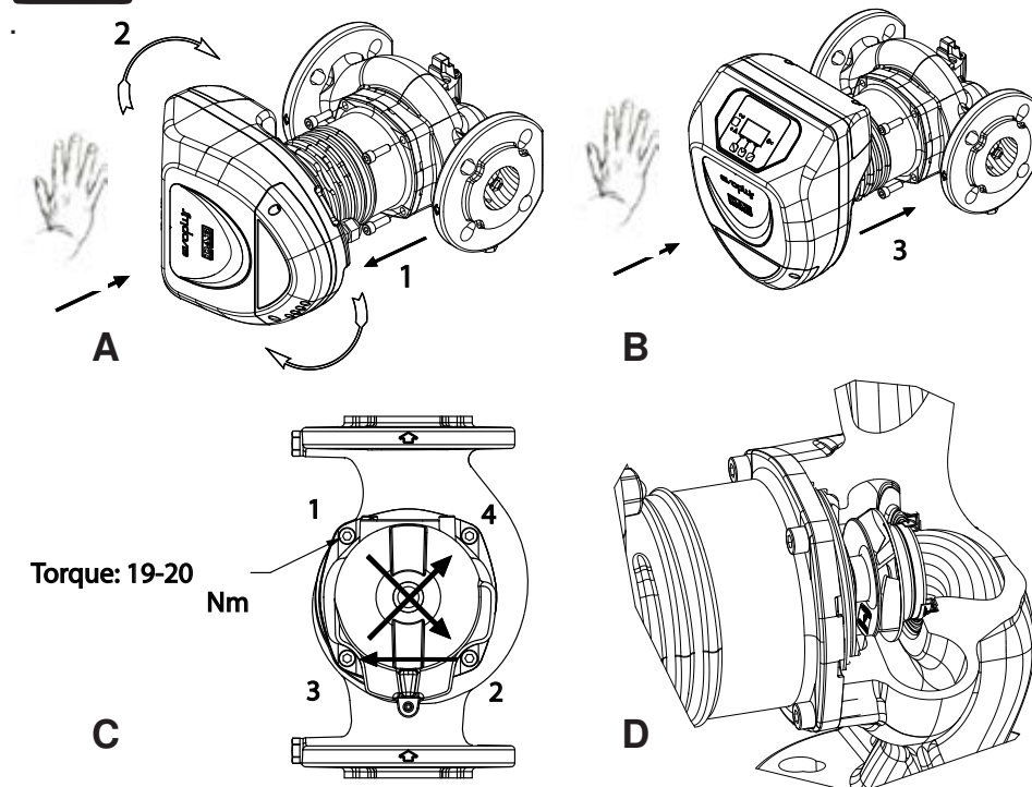
Figura 2: Instruções de montagem cabeças motor
