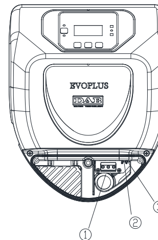
Attēls 4: Elektriskie savienojumi (priekšā)
