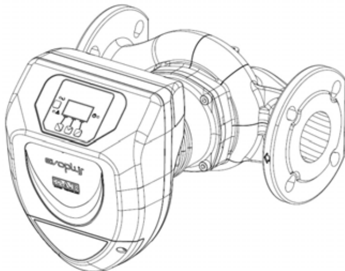
Afbeelding 3: Installatie op horizontale leidingen
