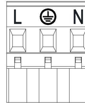
Figure 6 : Bornier d'alimentation amovible
