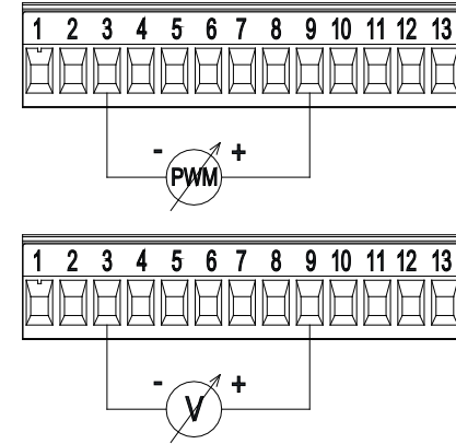
Attēls 8: Izņemams spaiļu panelis ar 13 kontaktiem: ieejas 0-10V un PWM
