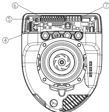
Εικόνα 5: Ηλεκτρική συνδεσμολογία (πίσω μέρος)
