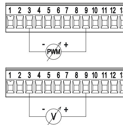
Figure 8 : Bornier amovible 13 pôles : entrées 0-10V et PWM
