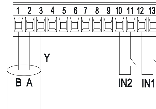
Figura 7: Morsettiera estraibile 13 poli: ingressi digitali e MODBUS
