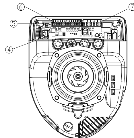
5 pav. Elektros jungtys (užpakalis)
