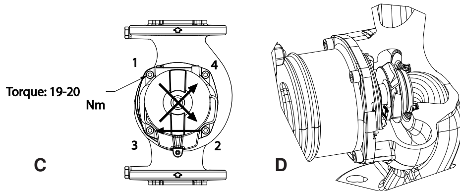
Сх 2: Инструкции по монтажу головок двигателя
