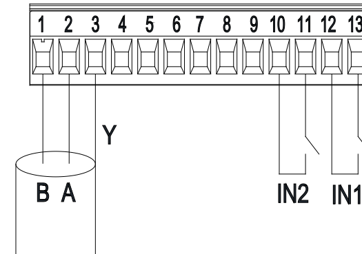
Figure 7 : Bornier amovible 13 pôles : entrées logiques et MODBUS
