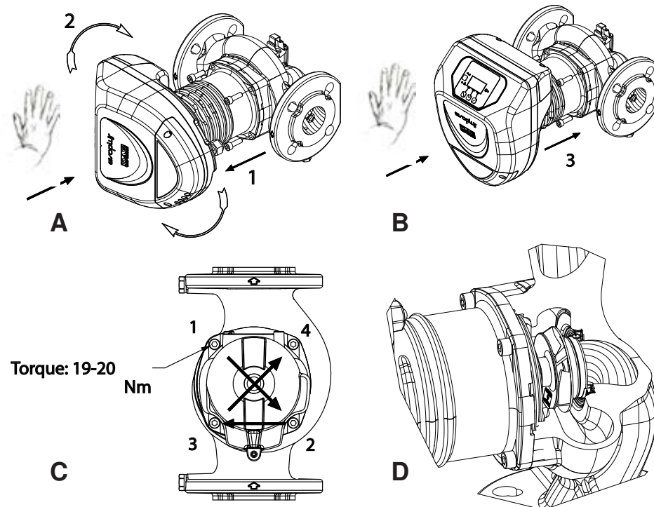
Фиг. 2: Инструкции за монтаж на моторната глава
