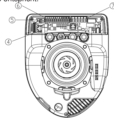
Abbildung 5: Elektroanschlüsse (Rückseite)
