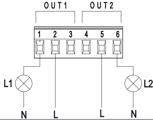
Resim 9: 6 kutuplu çekmeceli klemens kutusu: Çıkışlar bağlantı örneği
