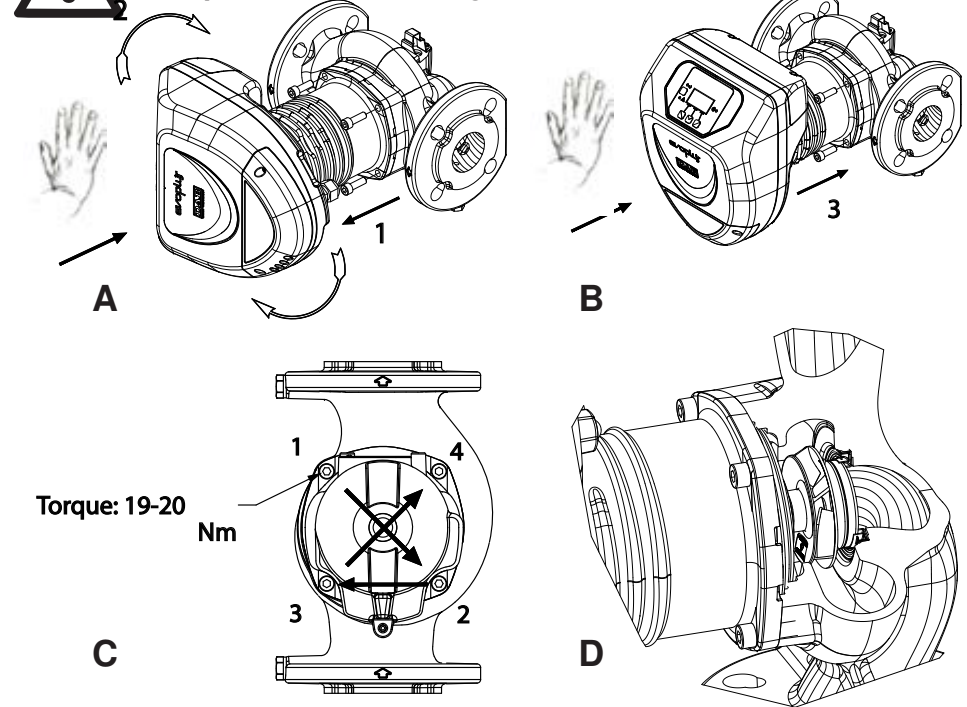
Figura 2: Istruzione di montaggio teste motore
