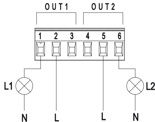
Εικόνα 9: Αφαιρούμενη κλέμμα 6 πόλων: παράδειγμα σύνδεσης εξόδων
