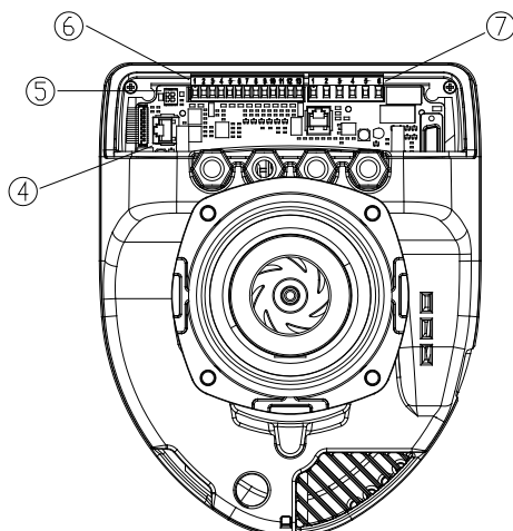
5. ábra: elektromos bekötések (háttoldal)
