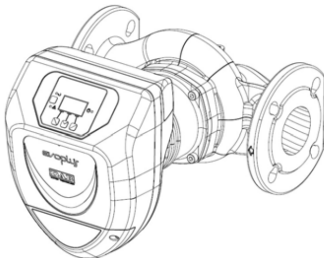
Slika. 3: Vgradnja na horizontalni cevi
