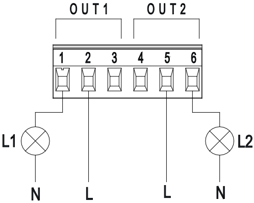
Figura 9: Terminal de bornes extraíble 6 polos: ejemplos de conexiones salidas
