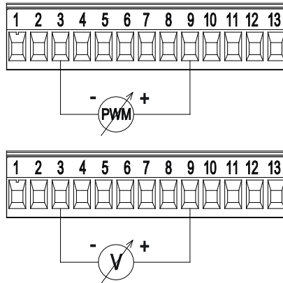
Εικόνα 8: Αφαιρούμενη κλέμμα 13 πόλων: είσοδοι 0-10V και PWM
