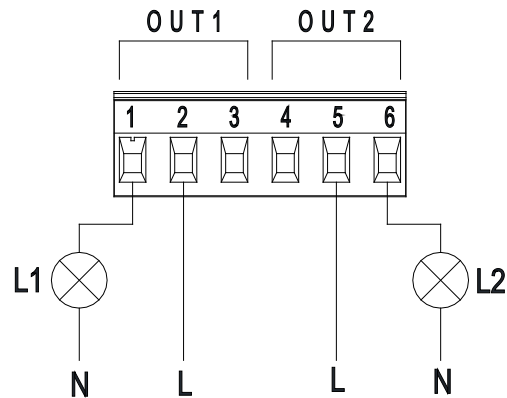
Afbeelding 9: Uittrekbare 6-polig klemmenbord: aansluitvoorbeeld van de uitgangen
