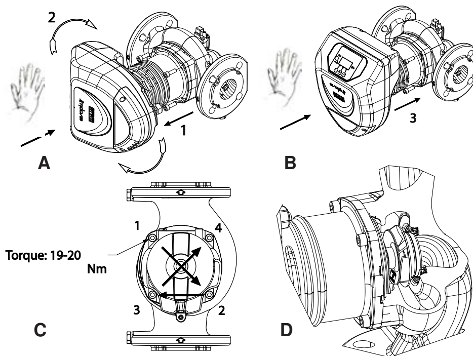
Obr. 2: Návod na montáž hláv motora
