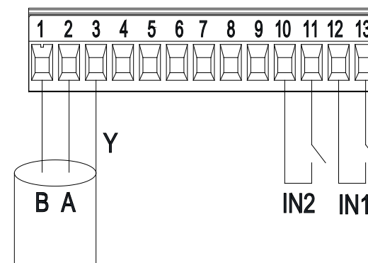
Εικόνα 7: Αφαιρούμενη κλέμμα 13 πόλων: ψηφιακές εισοδοι και MODBUS
