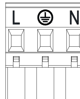
Obr. 6: Vyberateľná svorkovnica napájania
