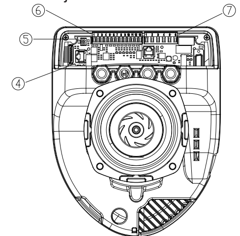
Attēls 5: Elektriskie savienojumi (aizmugurē)
