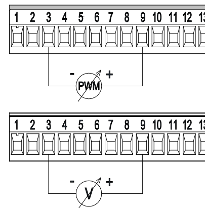
Figura 8: Morsettiera estraibile 13 poli: ingressi 0-10V e PWM
