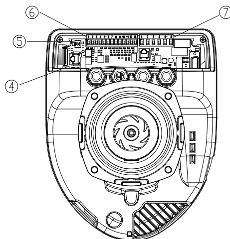
Figura 5: Conexiuni electrice (spate)
