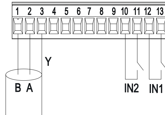
Afbeelding 7: Uittrekbaar 13-polig klemmenbord: digitale ingangen e MODBUS
