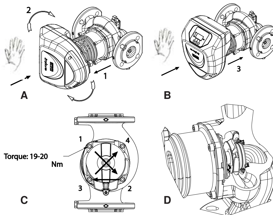
2 pav. Variklio galvučių įrengimo instrukcija
