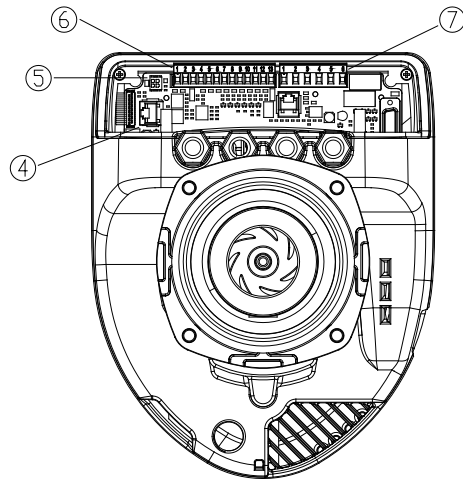
Afbeelding 5: Elektrische aansluitingen (achterzijde)
