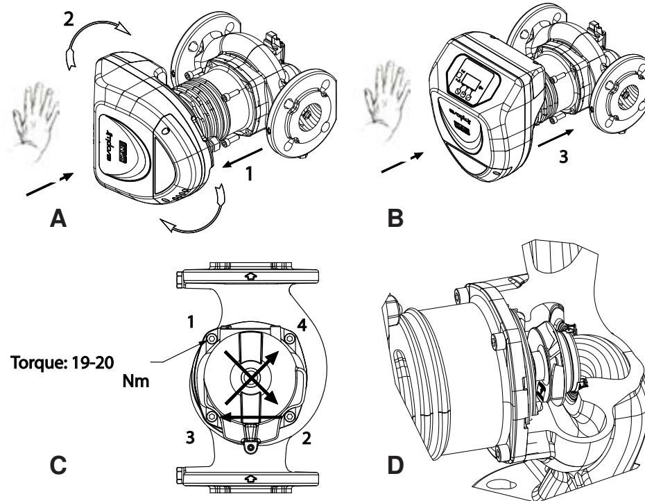
Kuv. 2: Moottorin päiden asennusohjeet
