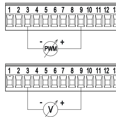
Afbeelding 8: Uittrekbaar 13-polig klemmenbord: ingangen 0-10V en PWM
