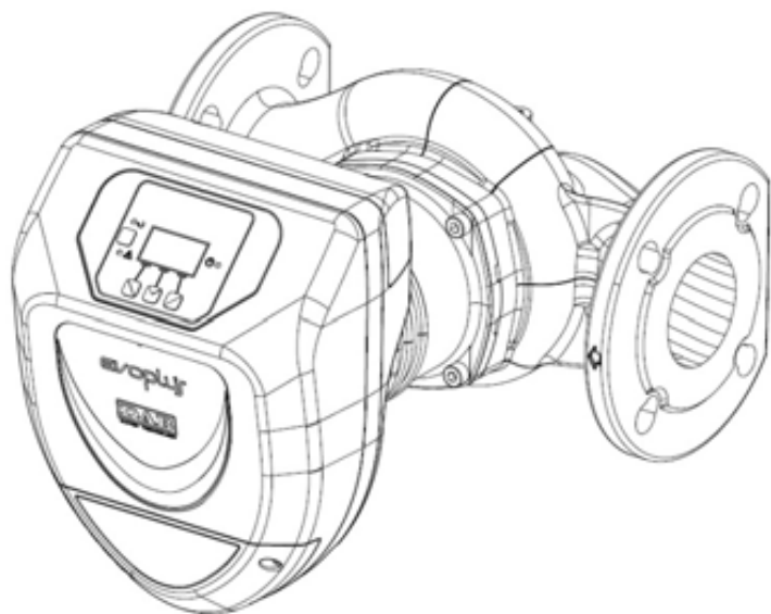
Rys. 3: Instalacja na przewodach poziomych
