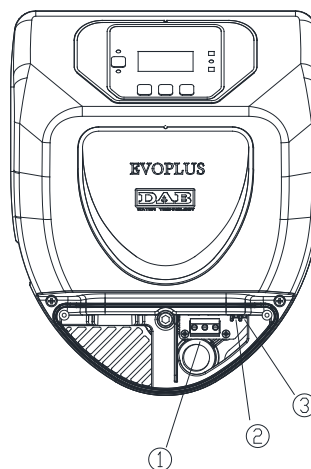
4 pav. Elektros jungtys (priekis)
