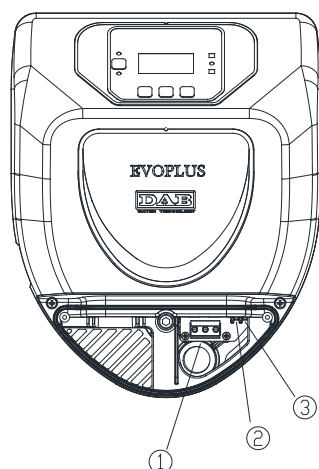
Figura 4: Conexiuni electrice (față)
