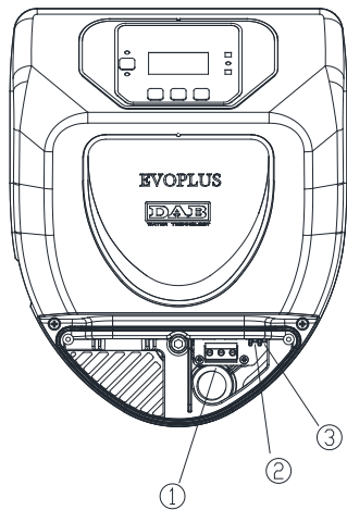
Figure 4 : Connexions électriques (face)
