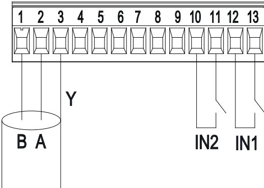
Attēls 7: Izņemams spaiļu panelis ar 13 kontaktiem: digitālās ieejas un MODBUS
