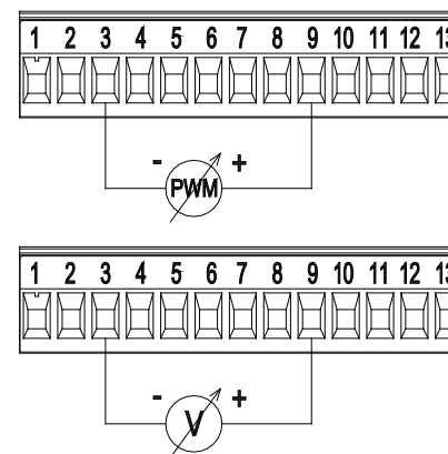
Fig. 8: 13-polig utdragbar kopplingsplint: Ingångar 0 - 10 V och PWM
