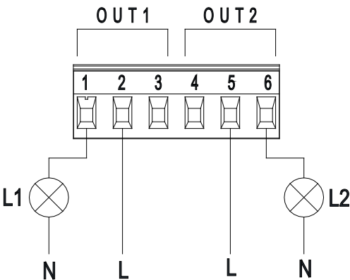
Figura 9: Barra de terminais extraível 6 pólos: exemplo de ligação das saídas
