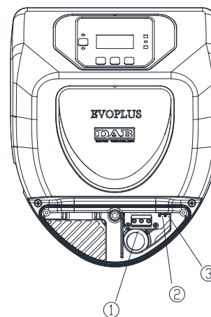
Figura 4: Connessioni elettriche(fronte)
