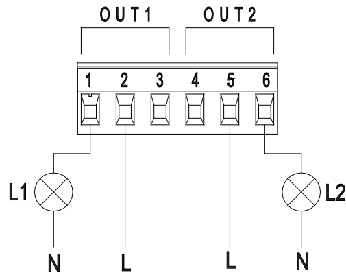
Figura 9: Morsettiera estraibile 6 poli: esempio di collegamento uscite
