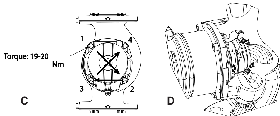
Figure 2: Instructions de montage têtes moteur
