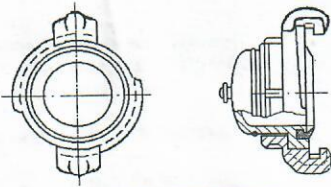
Рисунок – Головка-заглушка (рисунок не определяет конструкцию)
