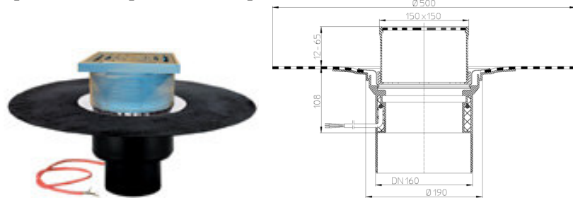
Рис. 3. Кровельная воронка с электрообогревом HL62.1BH/2.
