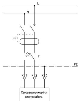
Рис. 5. Схема подключения электрообогрева кровельной воронки HL62.1BH к электрической сети.
