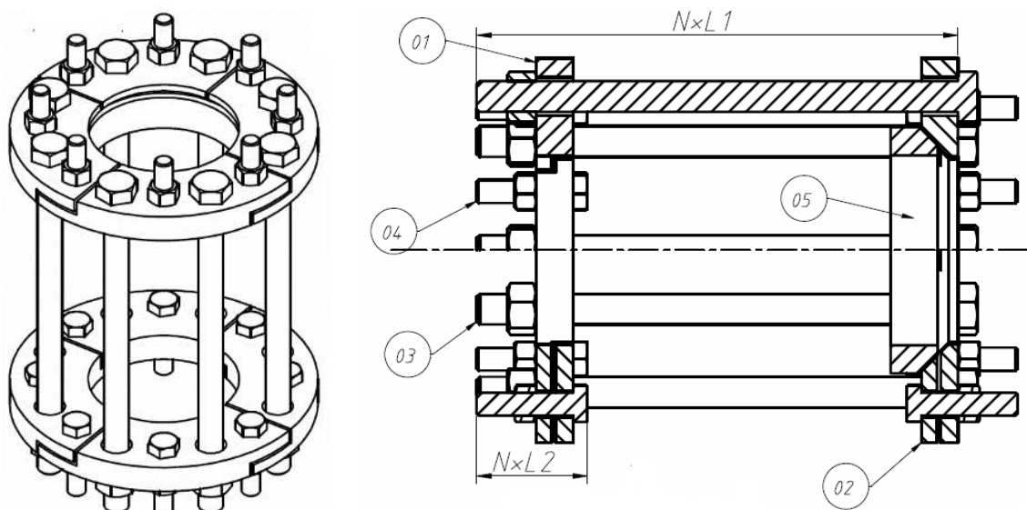
Рис.1. Ремонтное уплотнение раструбных соединений (РУРС).
