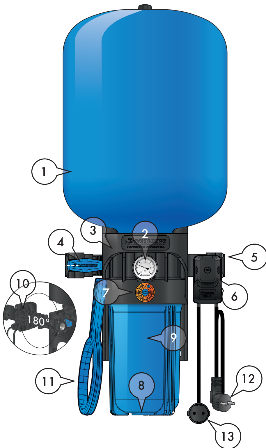
Рисунок 3 Схематическое изображение КРАБ-Т на примере КРАБ-Т 50
